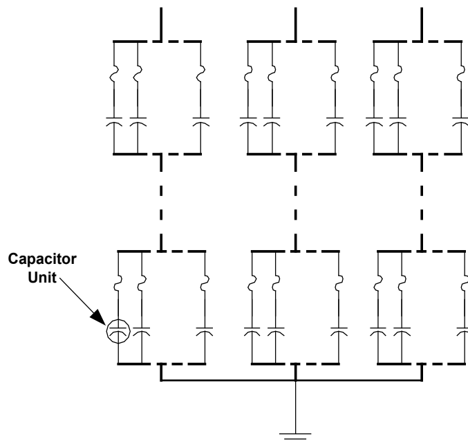
Figura 1b: Banco de Capacitores com Fusível Externo
