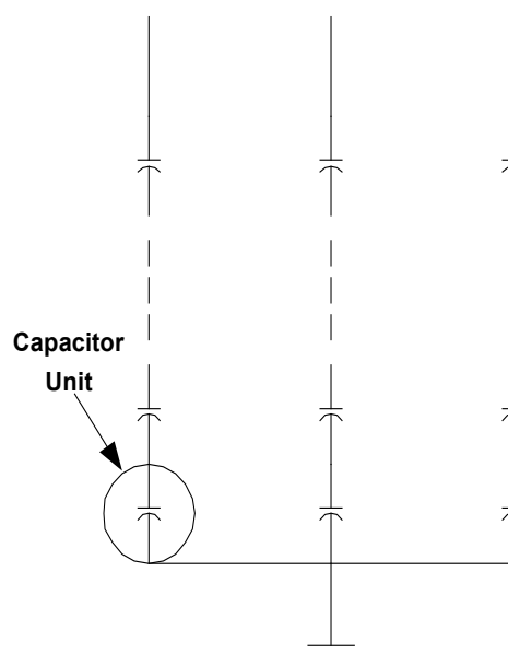
Figura 3b: Banco de Capacitores sem Fusível
