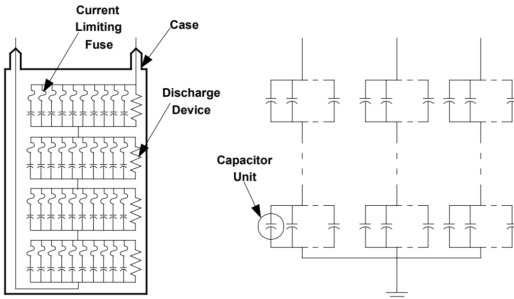
Figura 2a: Unidade Capacitiva com Fusível Interno
