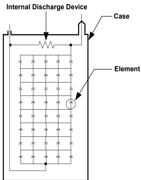
Figura 3a: Unidade Capacitiva sem Fusível
