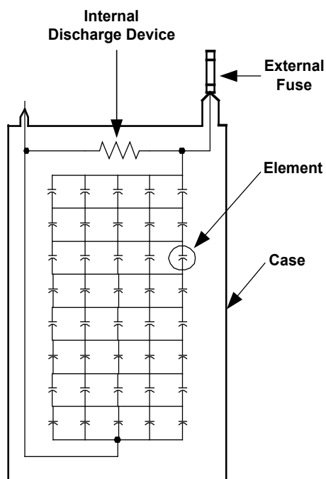
Figura 1a: Unidade Capacitiva com Fusível Externo
